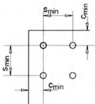
Anordnung Achs- und Randabstände
