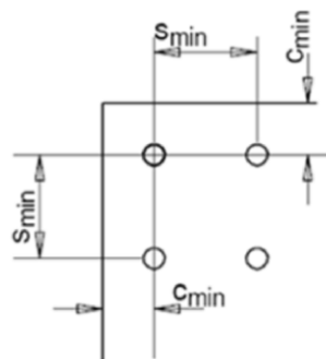
Schema der Achs- und Randabstände
