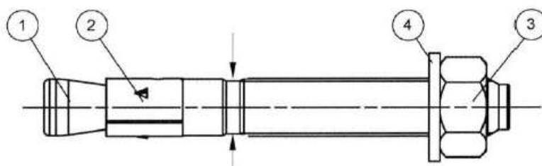
Trzpień stożkowy, wersja toczona:
