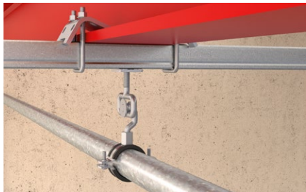
Binario su trave in acciaio.
