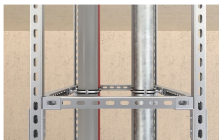
Telaio tridimensionale.
