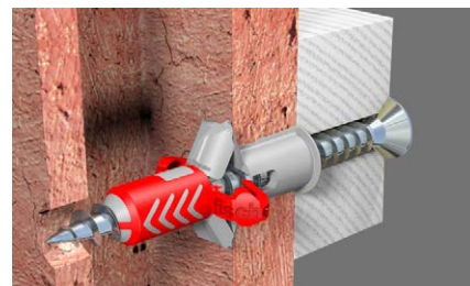
Installazione tasselli
