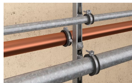
Fissaggio di tubazioni su profilo verticale.
