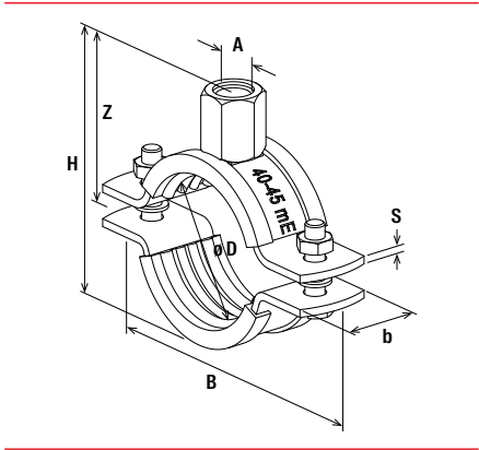
Collare pesante per tubi FRSM hdg
