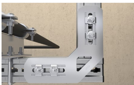
Dettaglio piastra di connessione.
