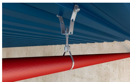
Installazione di sprinkler su lamiera grecata.
