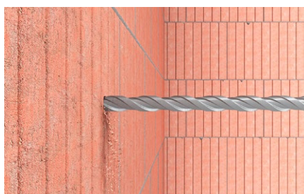
Foratura in mattoni forati
