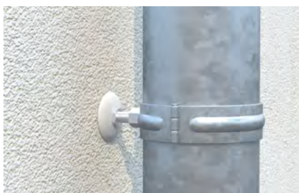
Fissaggio di collari per tubi pluviali su sistemi compositi di isolamento termico esterno (ETICS)
