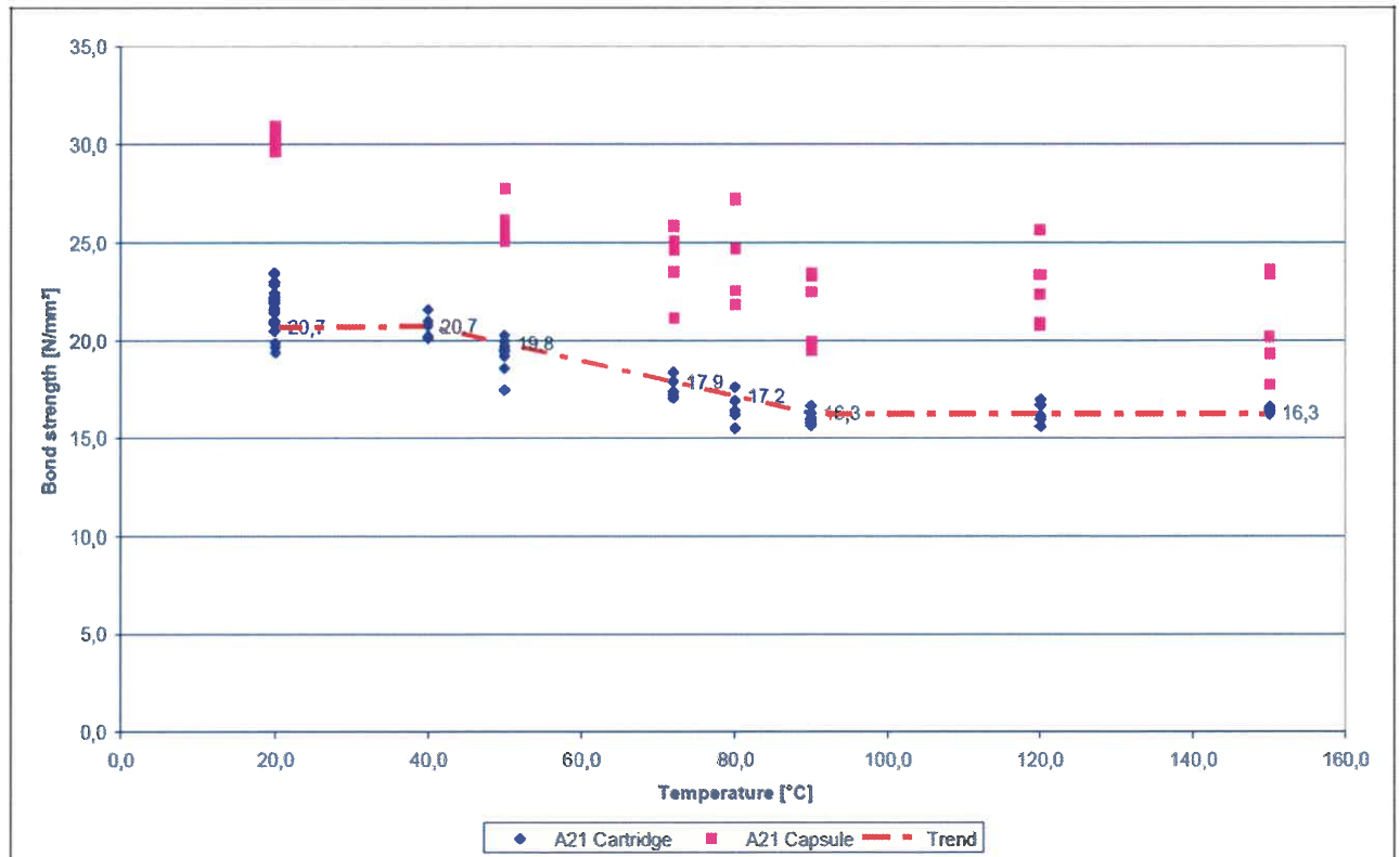
Bild 1: Vergleich der Verbundspannungen in Abhängigkeit der Temperatur zwischen „FIS SB“ und „RSB“
