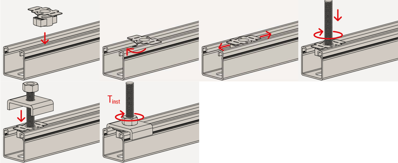
Bild B 3.1 – Montageanleitung der Schiebemutter FCN Clix P
