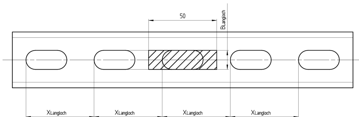
Bild B 5.1: Parameter für die Berechnung des gemittelten Querschnittsprofils
