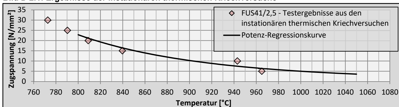
Bild D 2.1: Ergebnisse der instationären thermischen Kriechversuche
