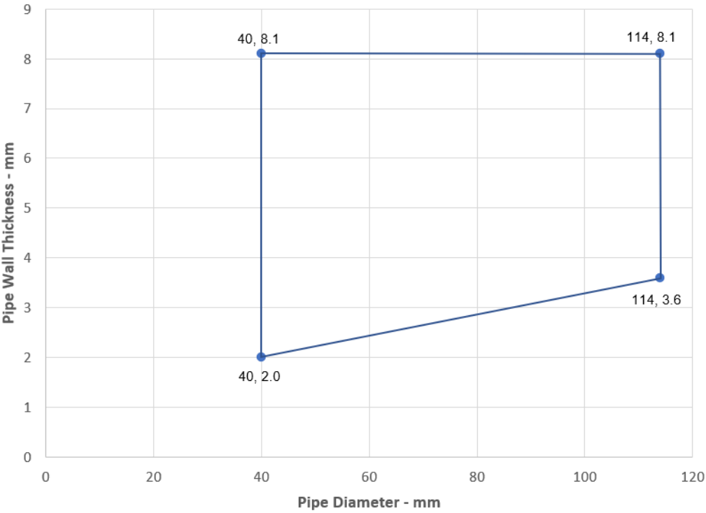
PE Pipes - EI 60 U/C
