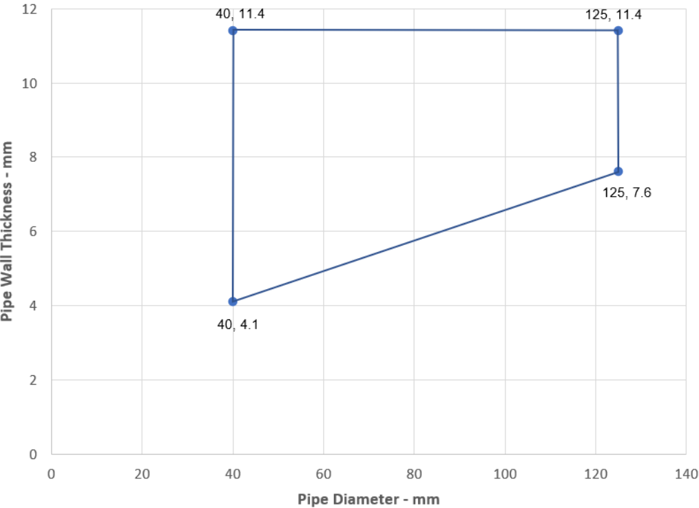
PE Pipes - EI 60 U/C
