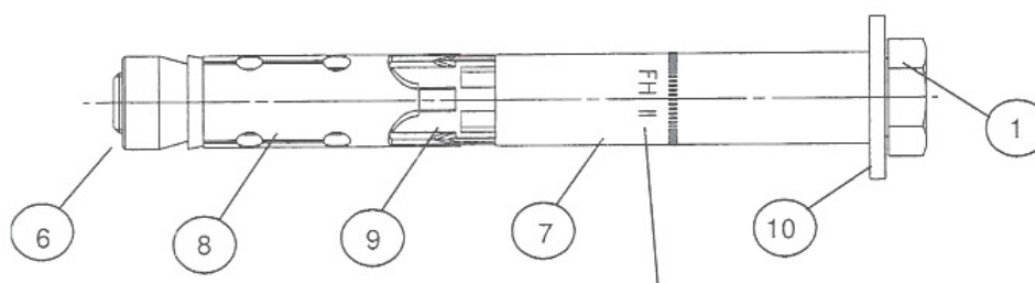
Version avec vis Type S FH II 10 - 32
