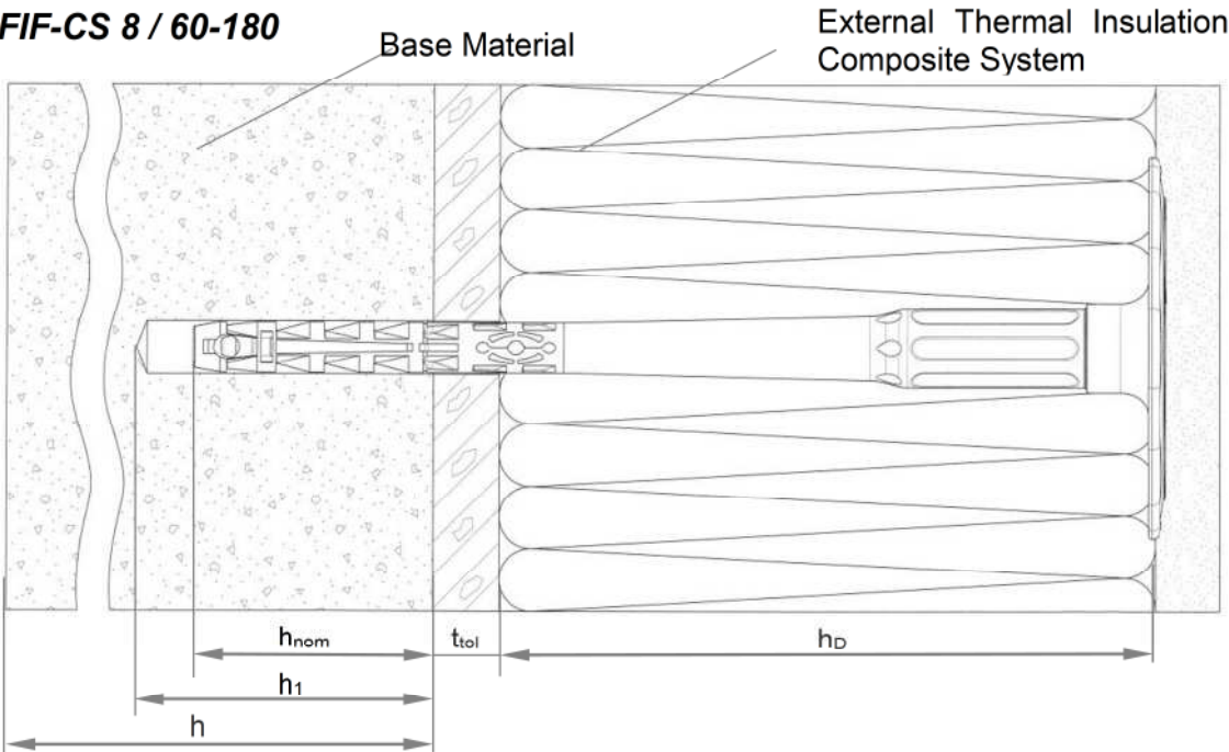
FIF-CS 8 / 200-340
