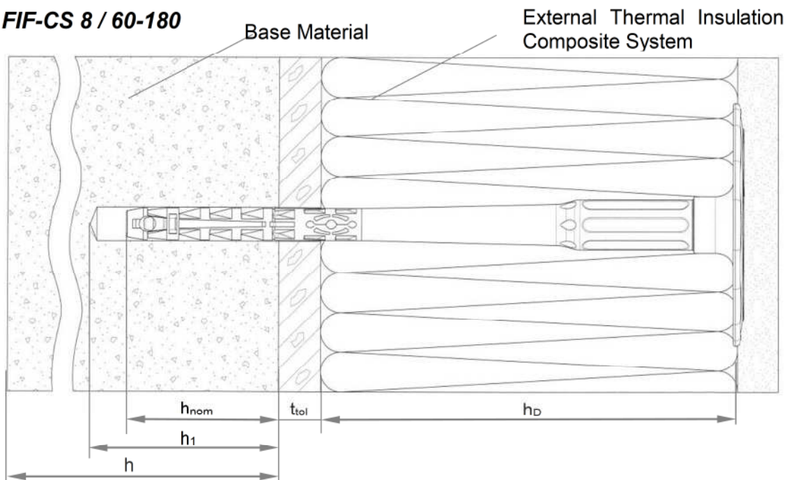
FIF-CS 8 / 200-340
