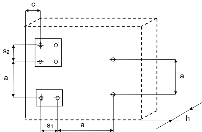
Anordnung der Achs- und Randabstände in Beton, Verankerungsgrund Gruppe „a“
