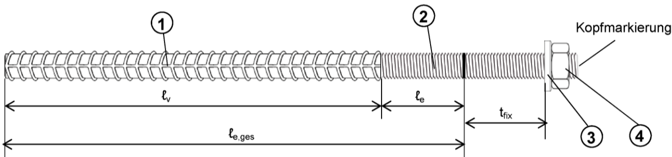
Bild A10: Eigenschaften von Upat Bewehrungsankern
